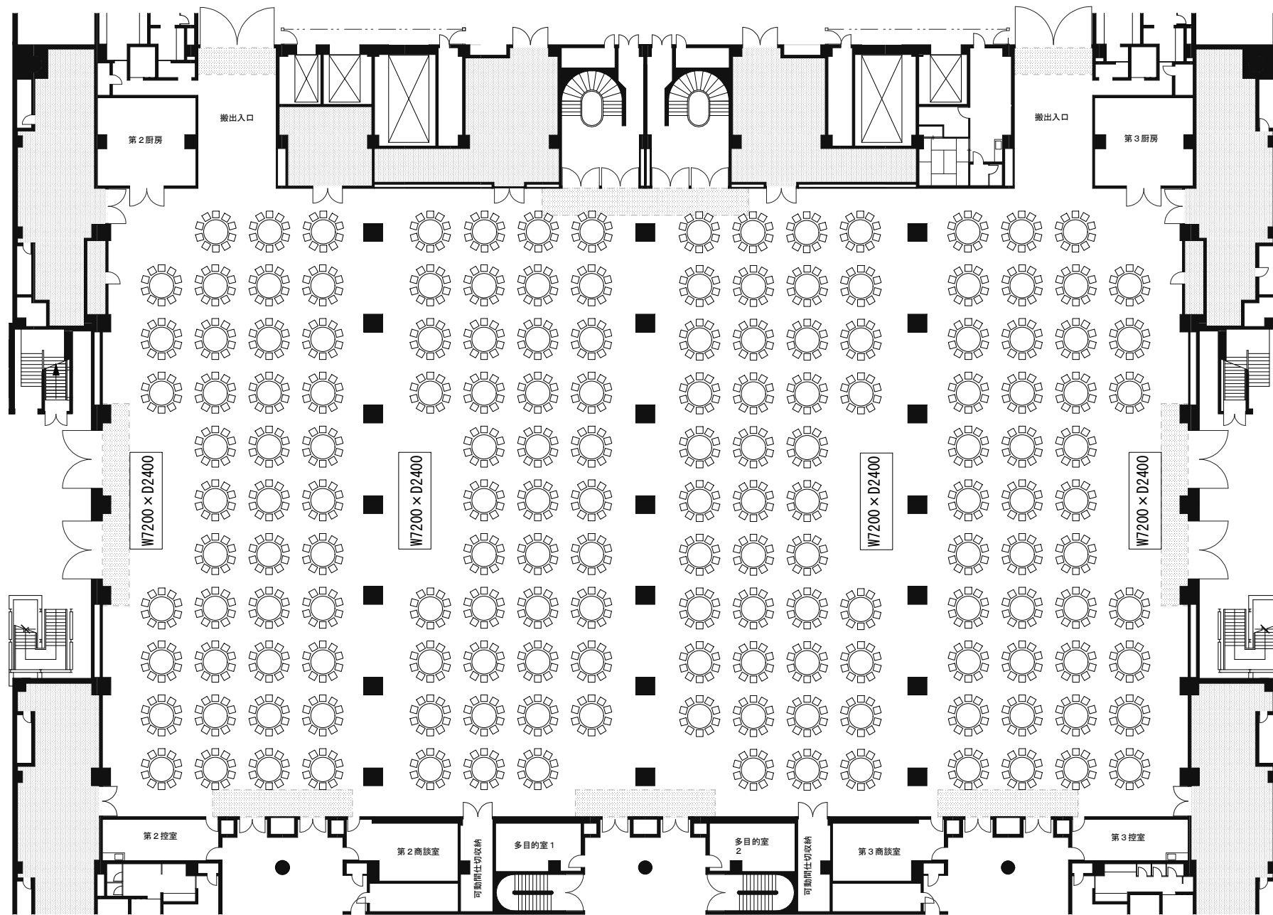
1卓10名×40卓：400席
