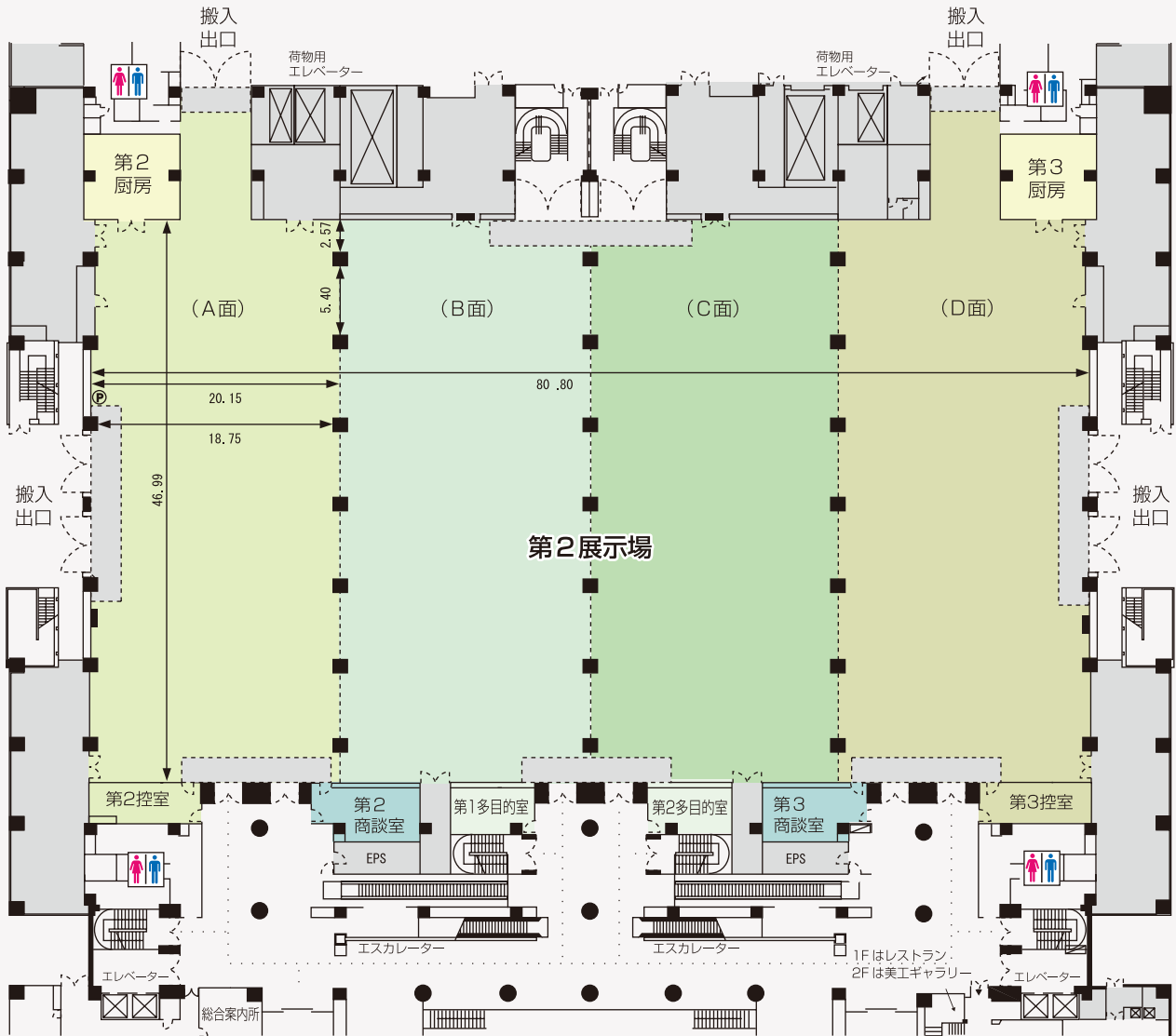
第2展示場柱寸法
